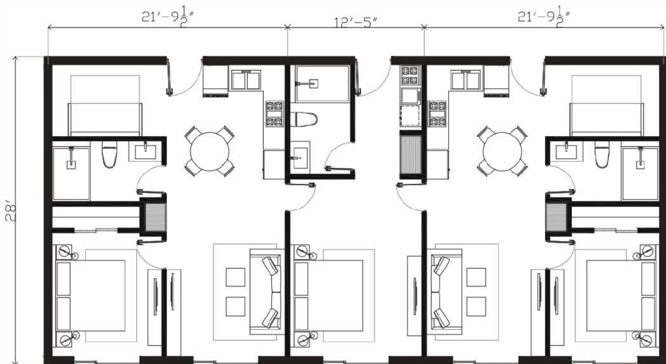
SUITE ONE BEDROOM + DEN
